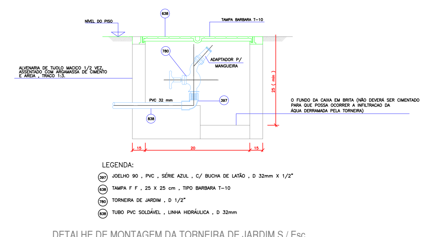
DETALHE DE MONTAGEM DA TORNEIRA DE JARDIM S / Esc.
